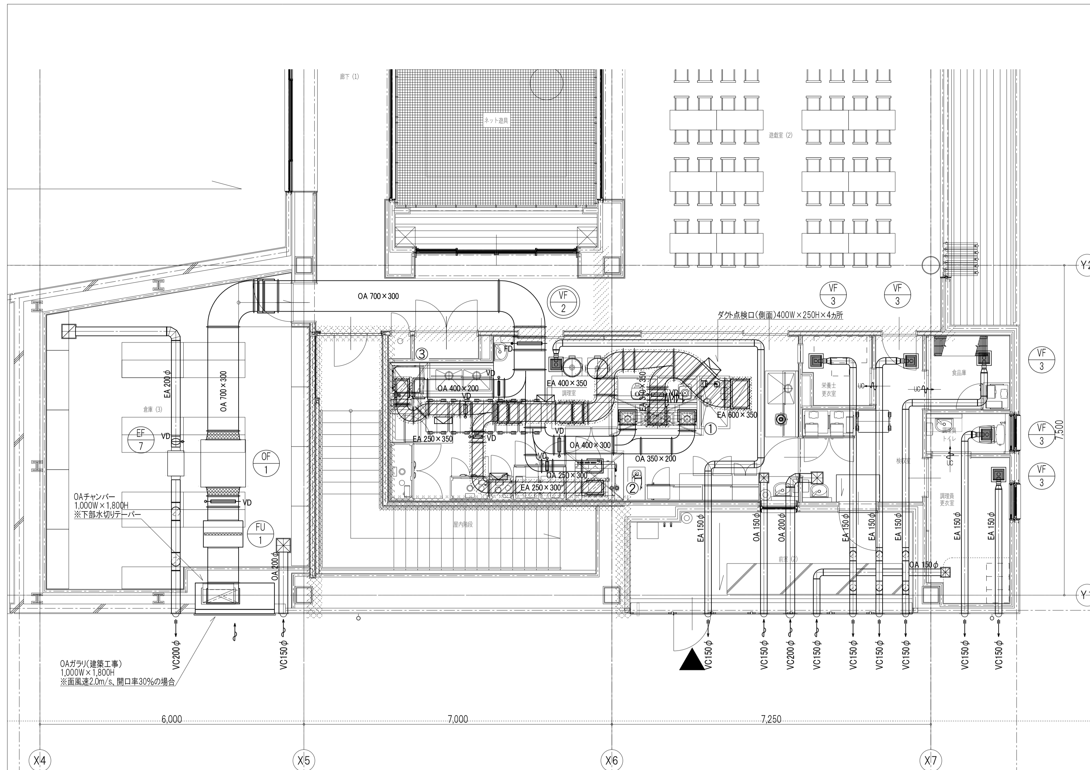
1階ダクト詳細図
