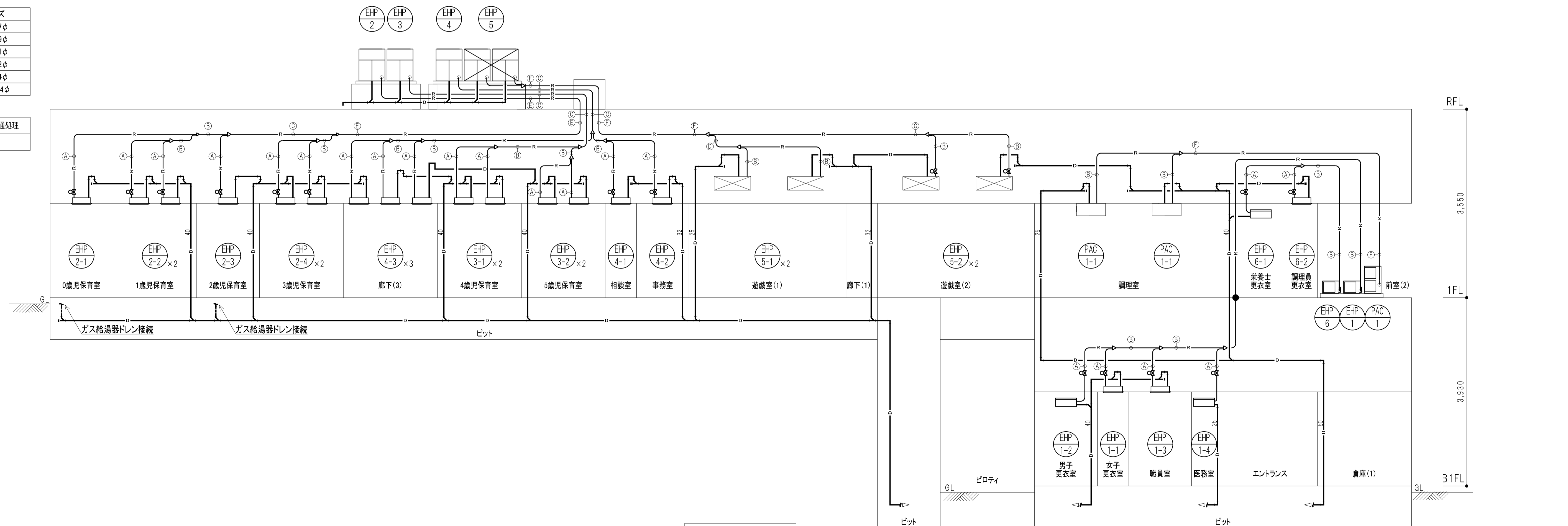
配管系統図
