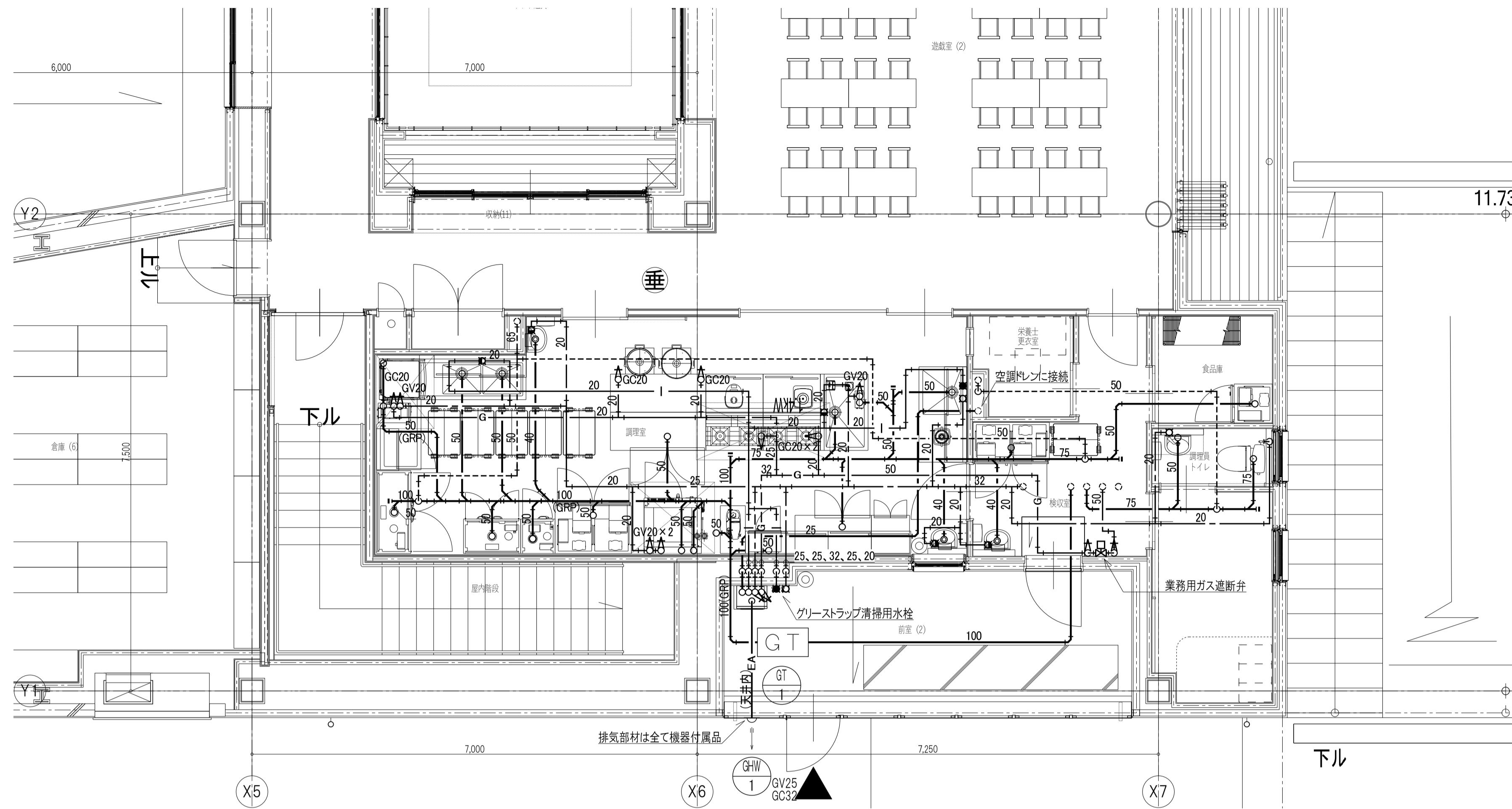
1階詳細図(1)
