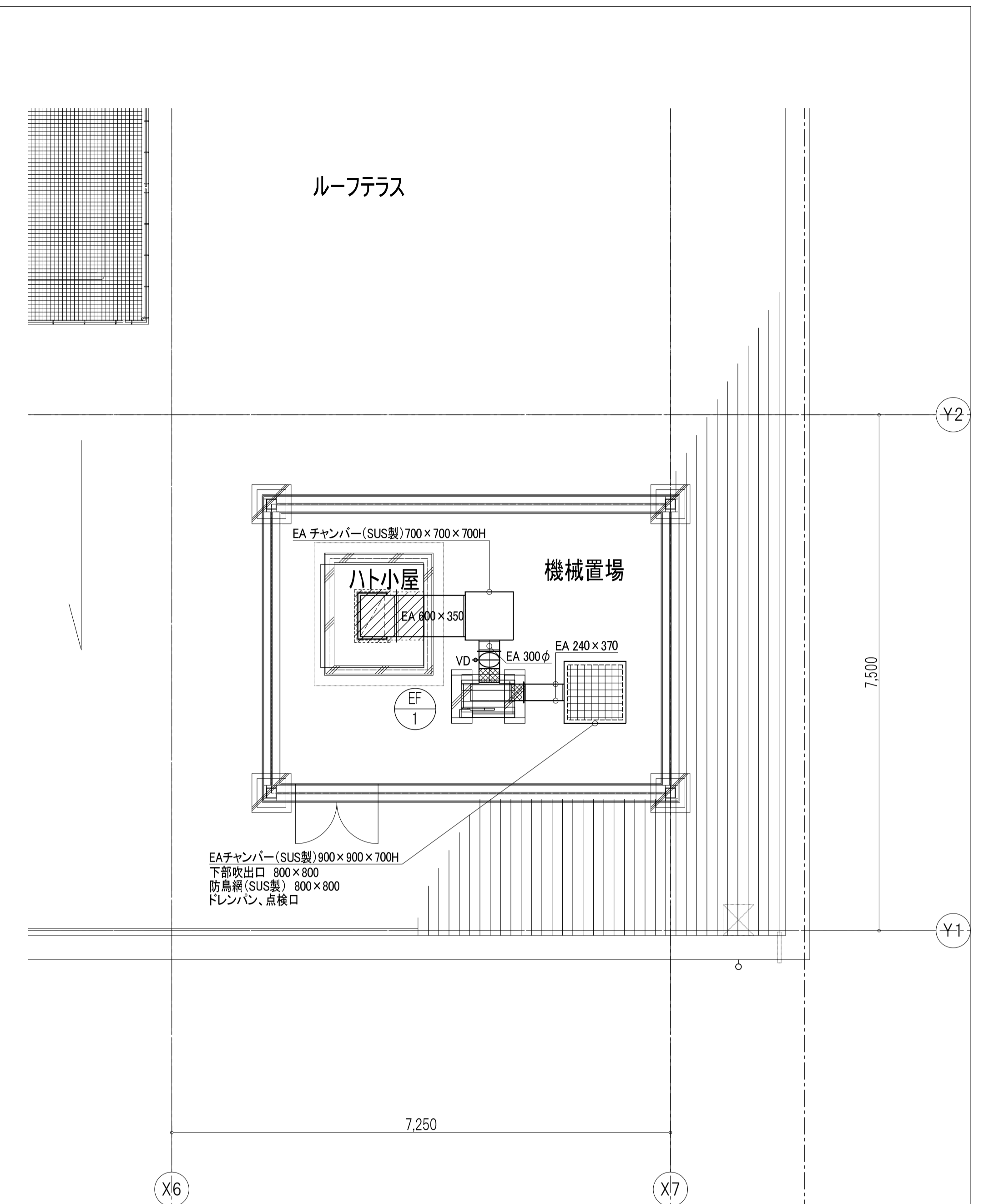
屋上ダクト詳細図
