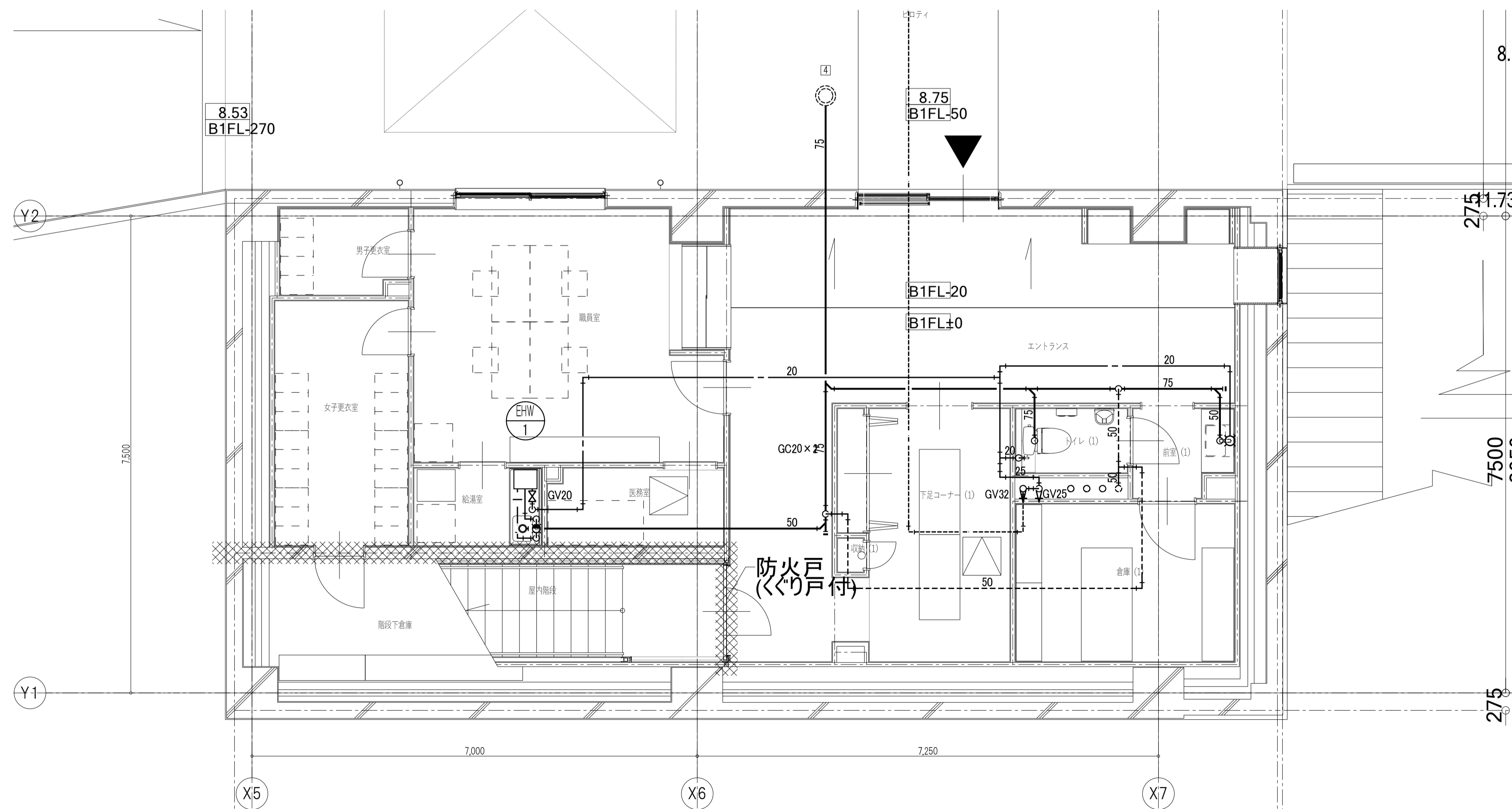
地下1階詳細図
