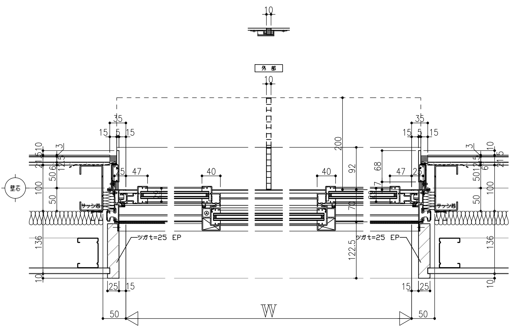
平面図 (腰窓)
