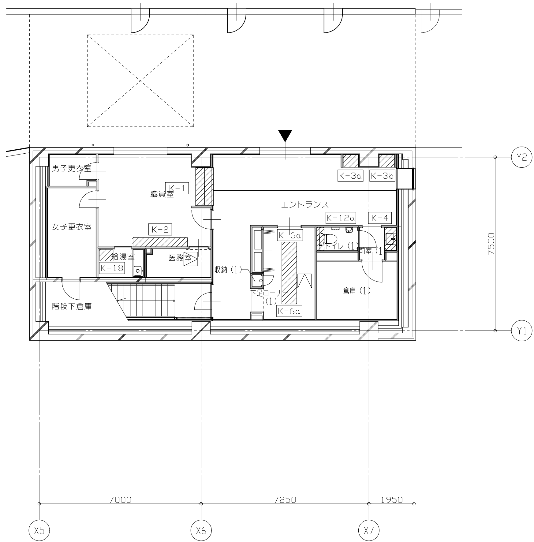
地下1階平面図
