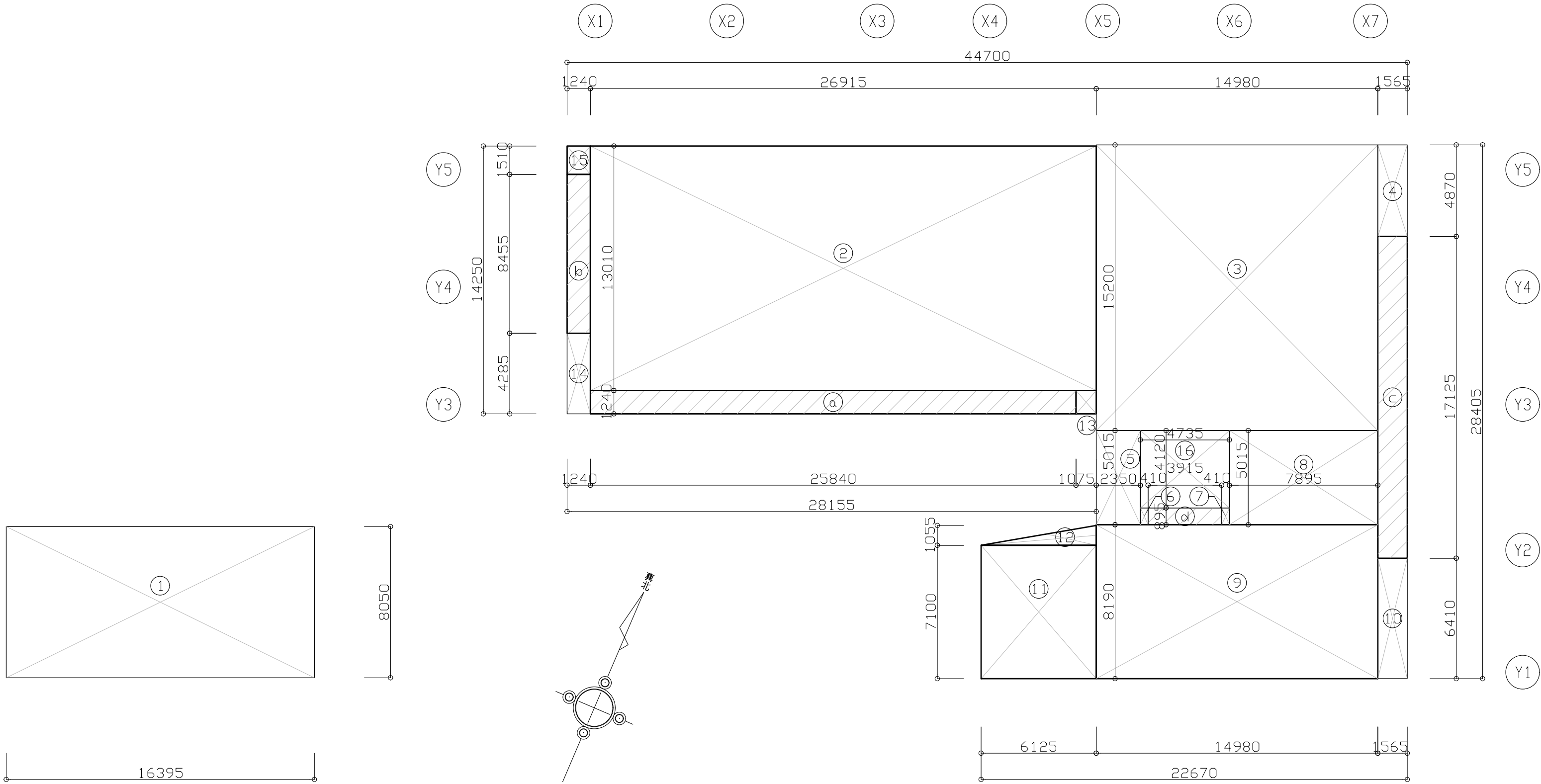
地下1階建物求積図
