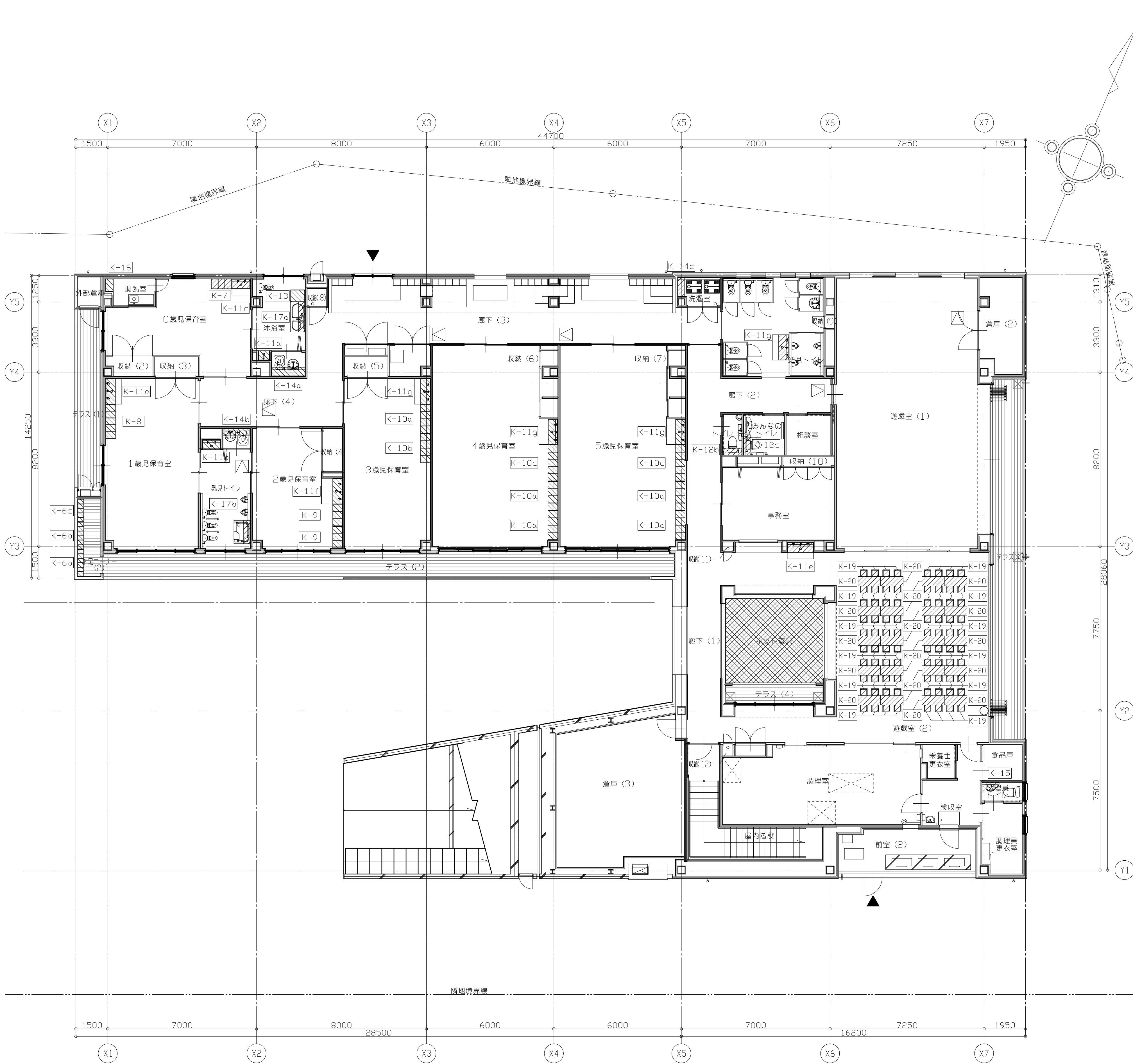
1階平面図
