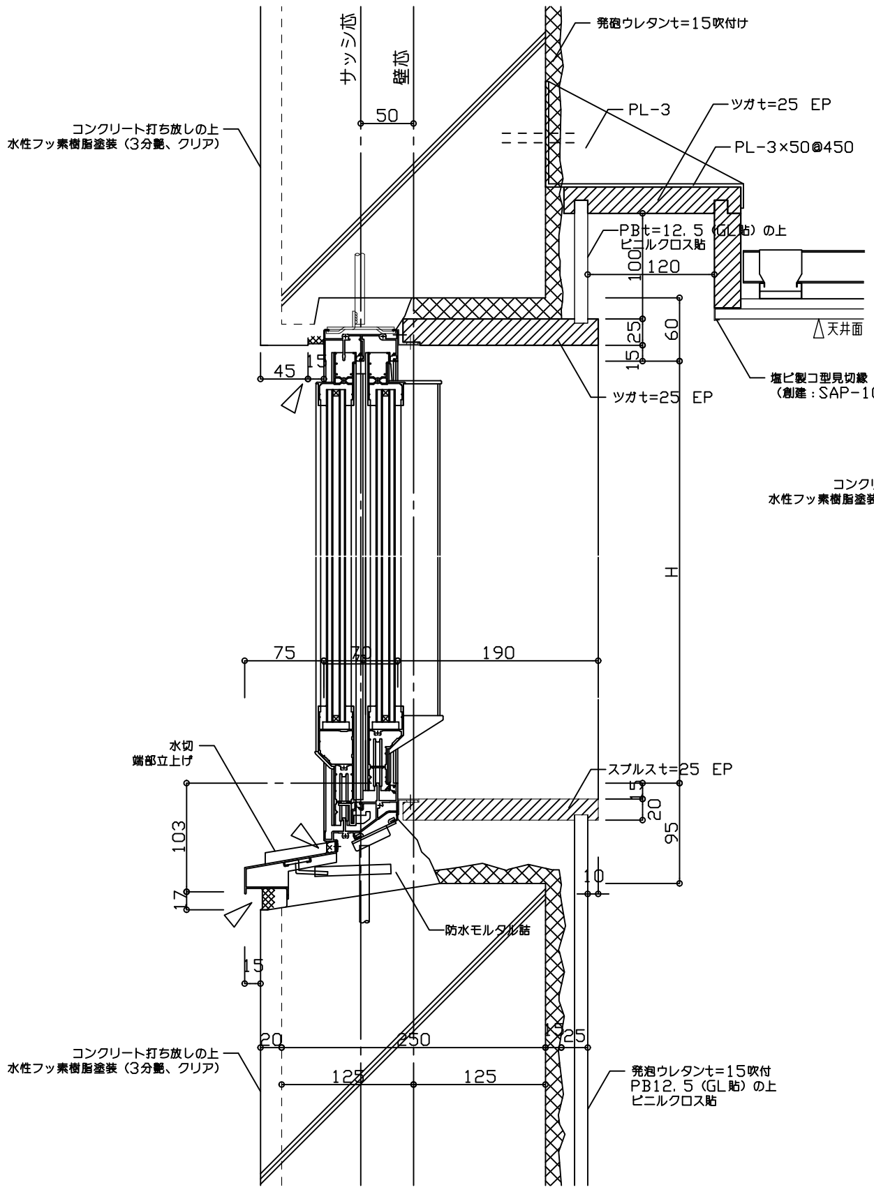
断面図 (RC 躯体腰窓)
