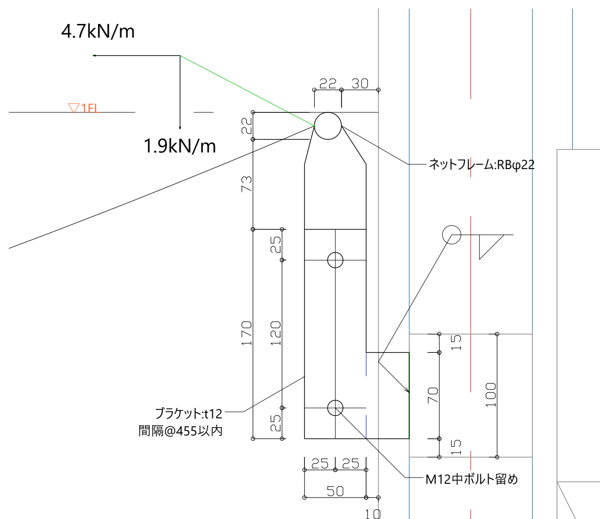
ネットフロア1層目ラッキングバー標準図
