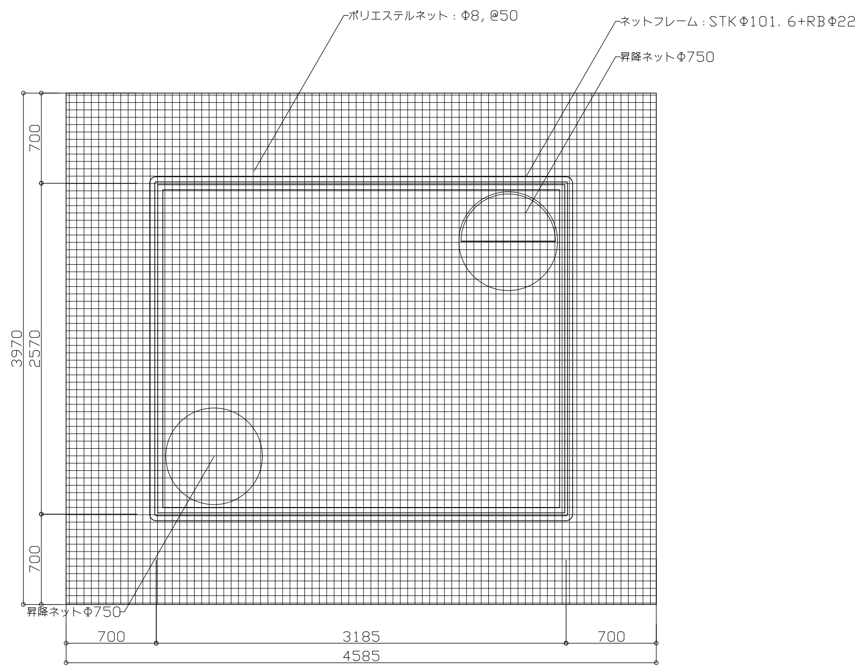
ネットフロア2層目(1FL+2250) 平面図
