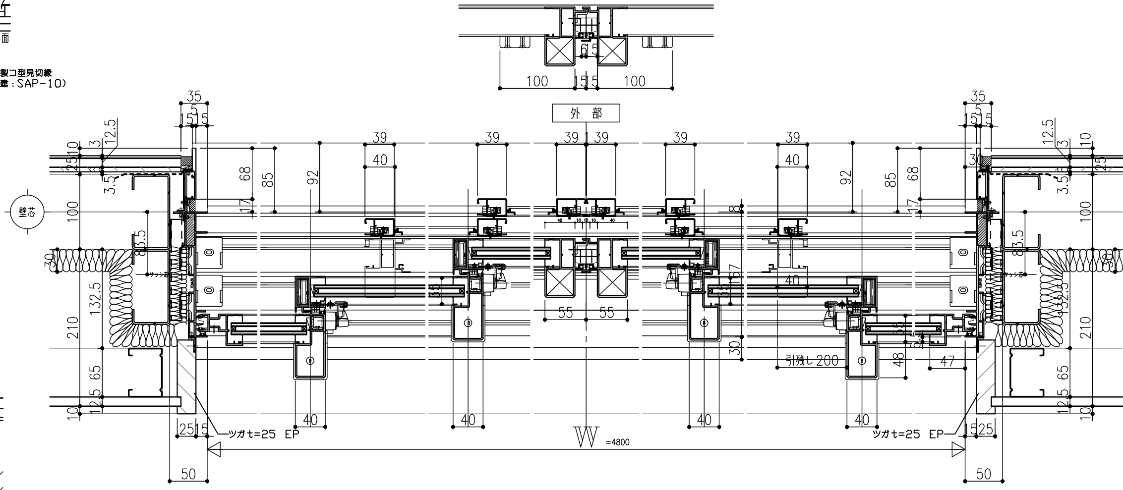
平面図 (6枚建て掃き出し窓)
