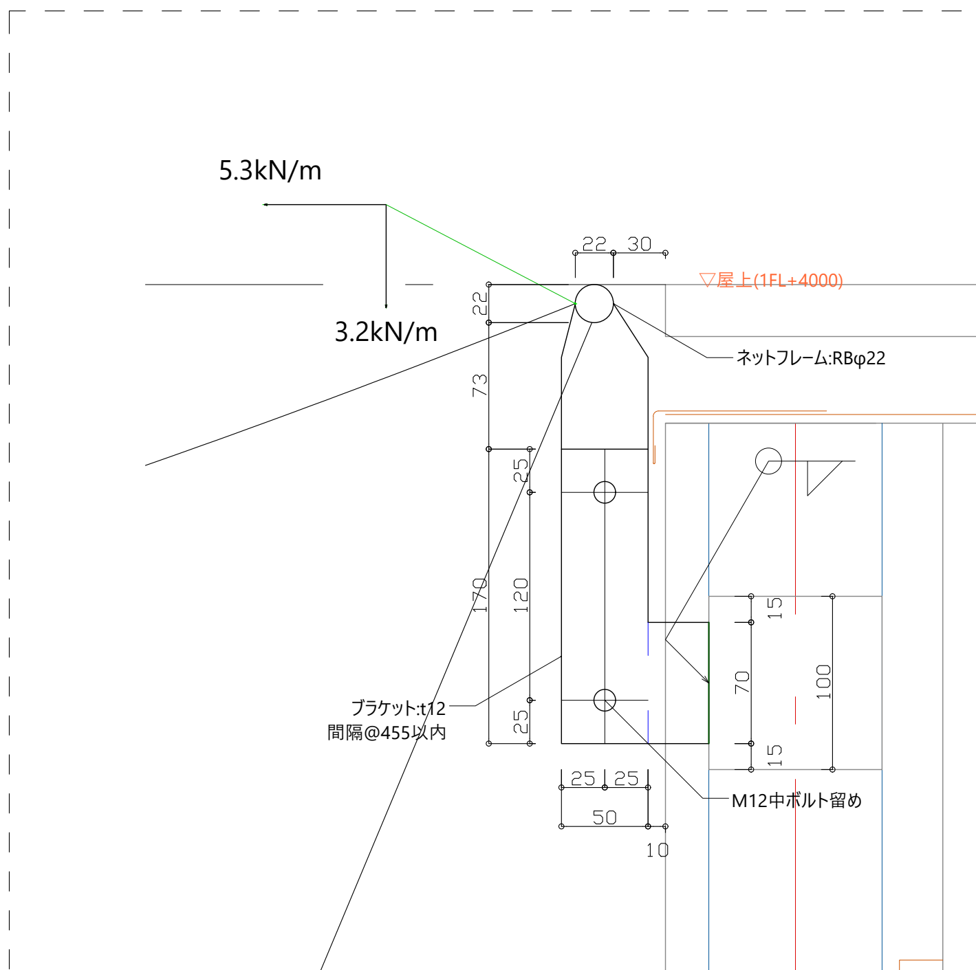
ネットフロア3層目フレーム取付部側面図 S=1: 15
