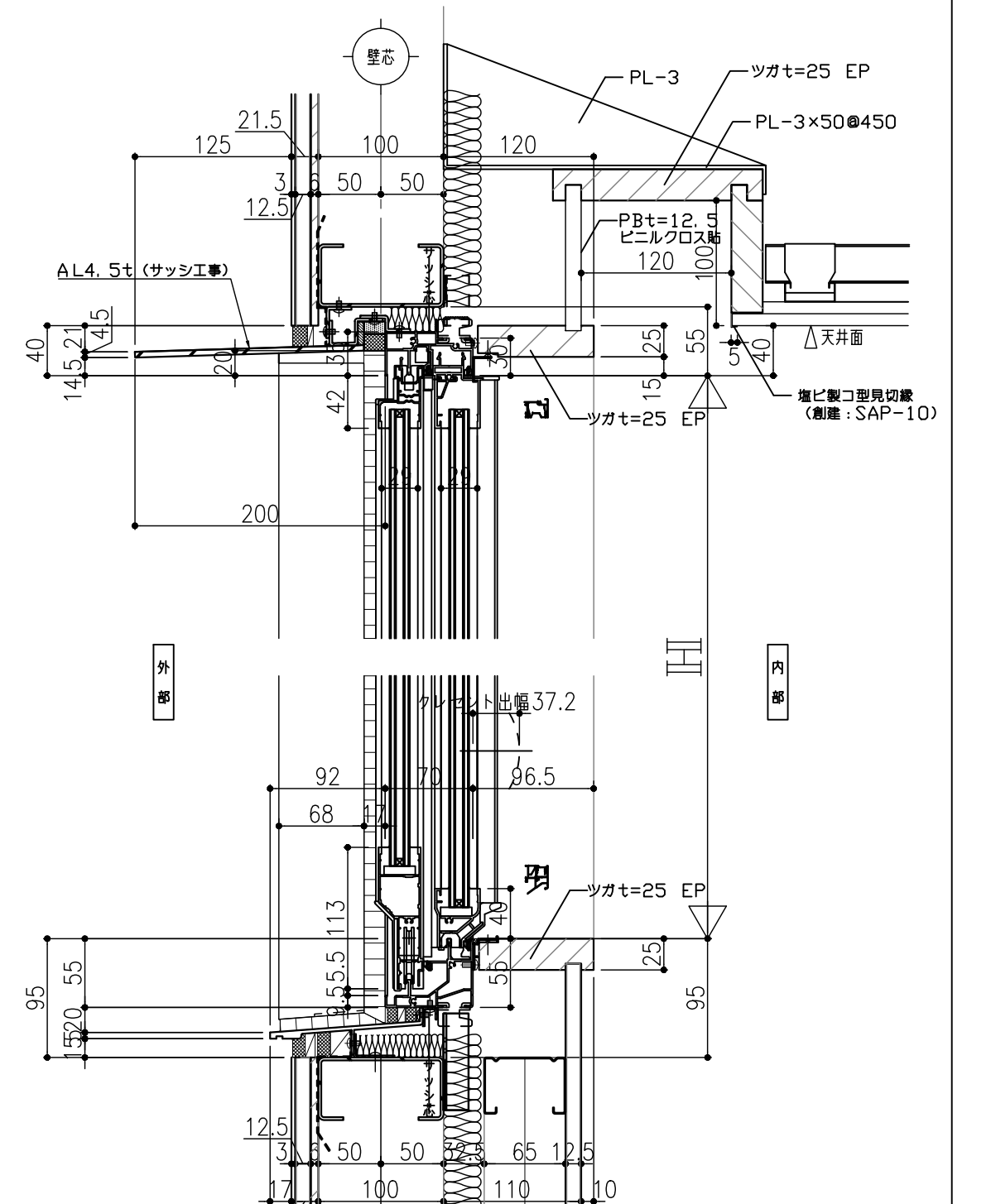
断面図 (腰窓)
