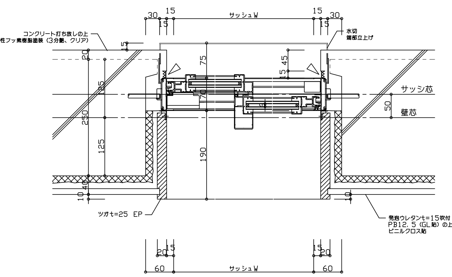
平面図 (RC 躯体腰窓)
