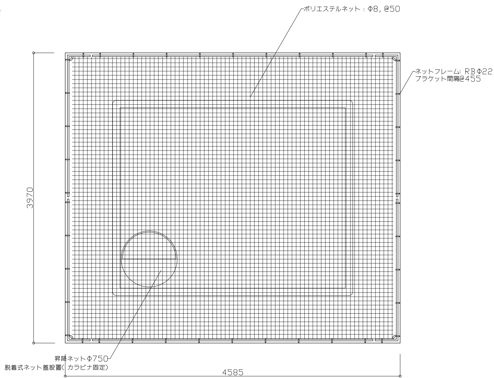
ネットフロア3層目(1FL+3950) 平面図
