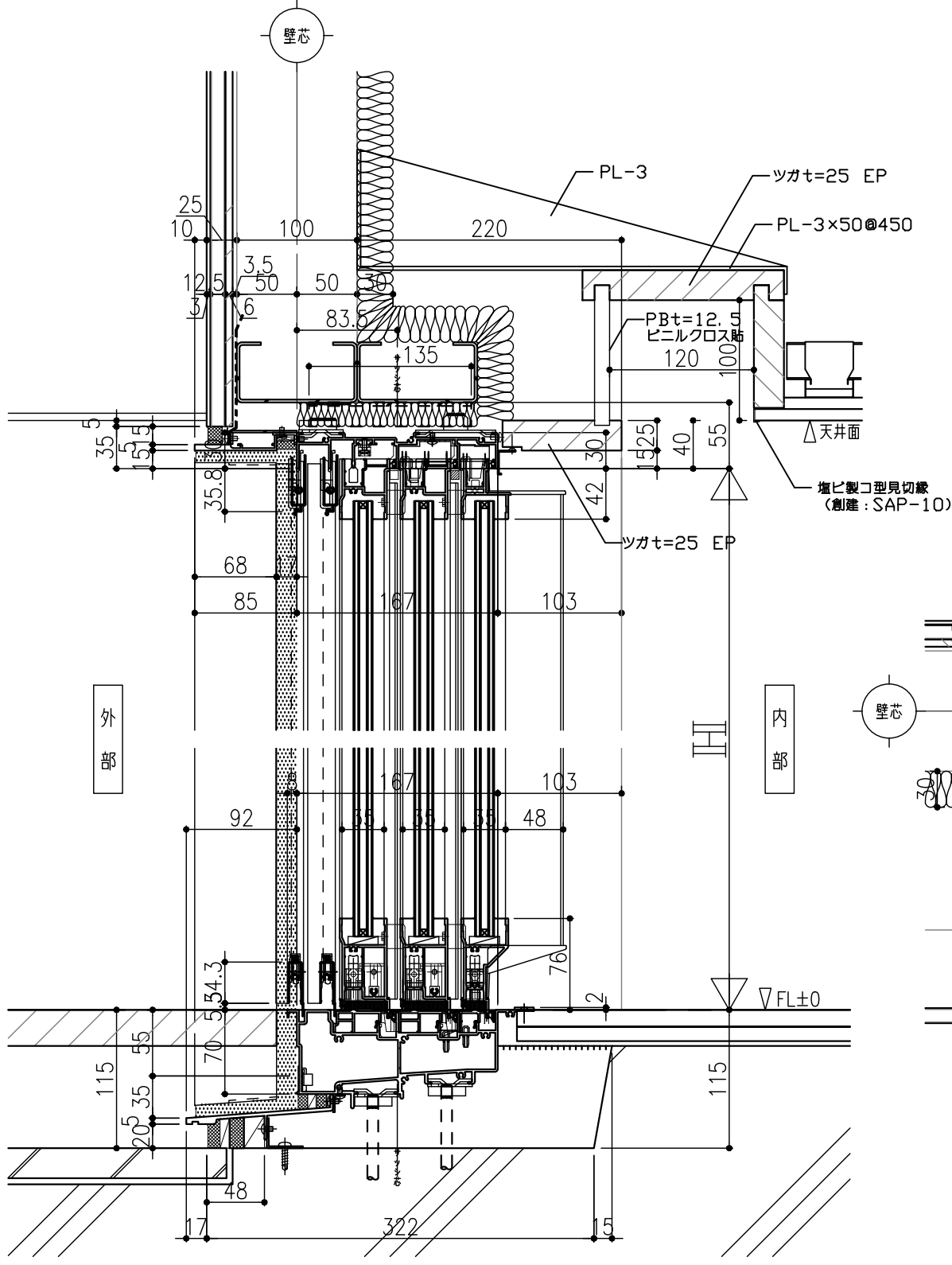
断面図 (6枚建て掃き出し窓)
