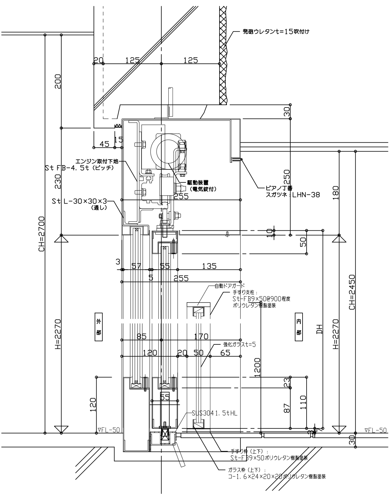
断面図
