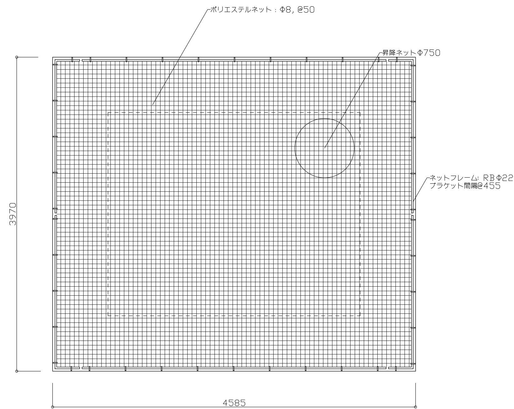
ネットフロア1層目(1FL±0) 平面図
