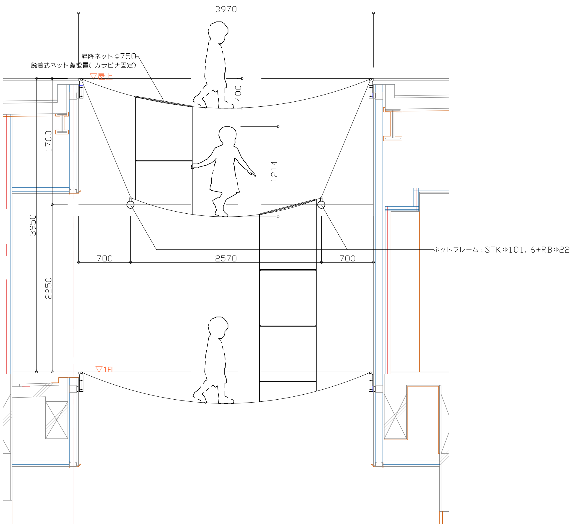
断面図
