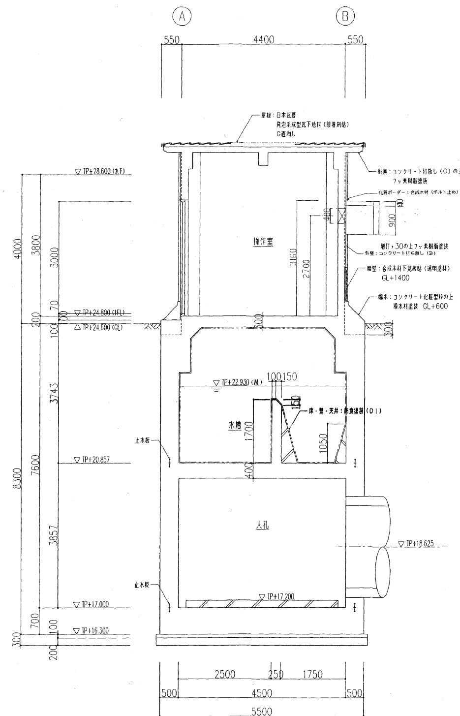
B-B 断面詳細図 S=1/50
