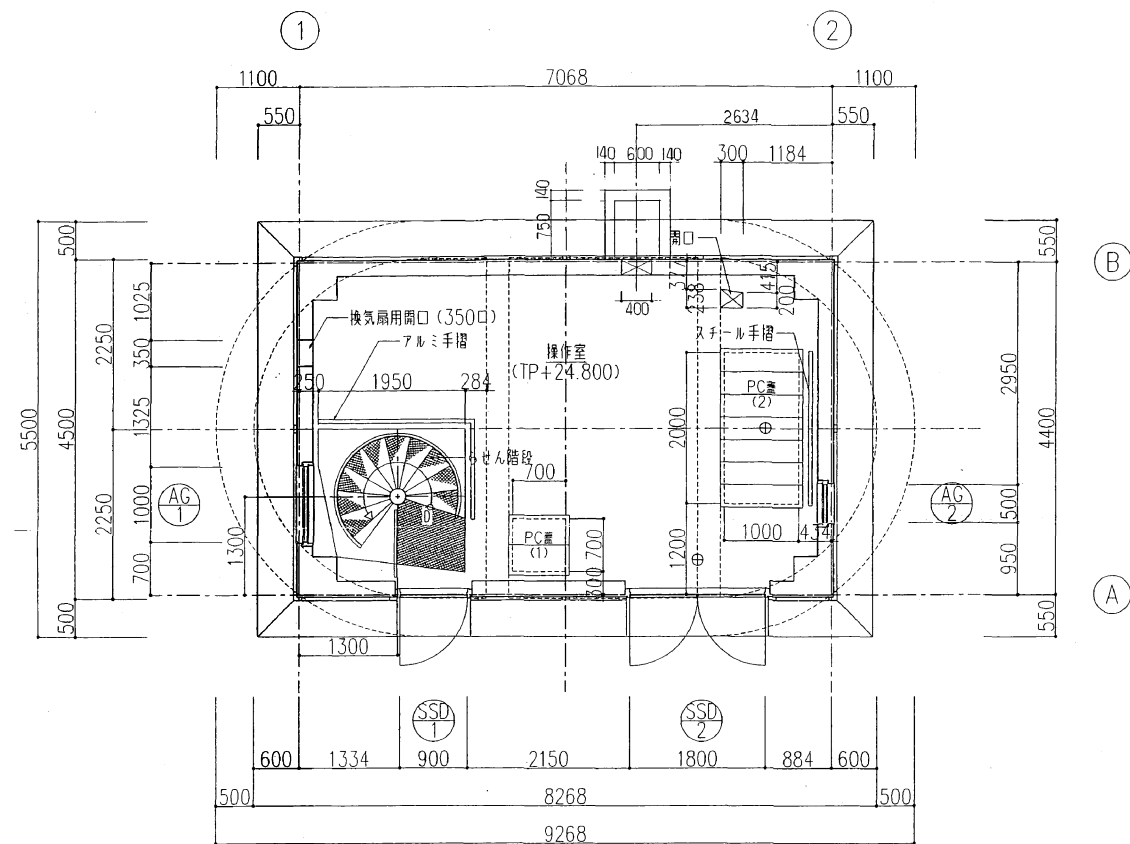
1階平面詳細図 S=1/100
