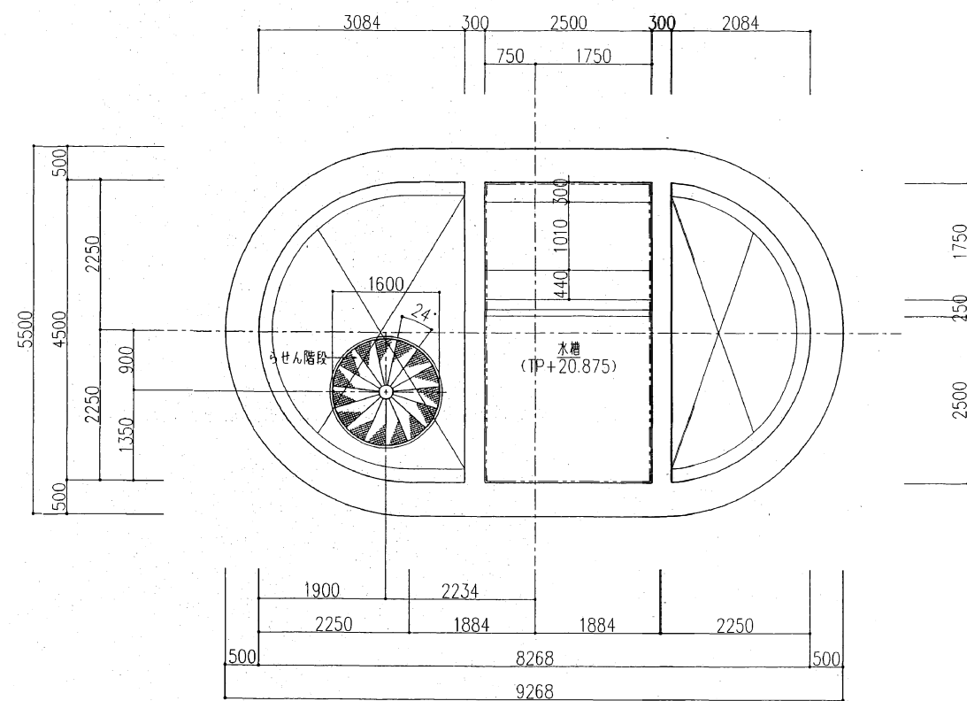
TP+20.875 平面詳細図 S=1/100
