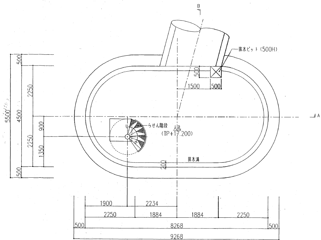
TP+17.000 平面詳細図 S=1/100
