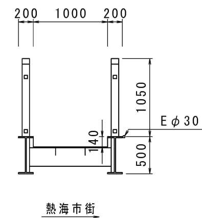
断面図
