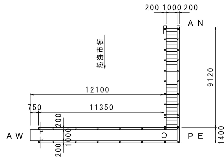
平面图
