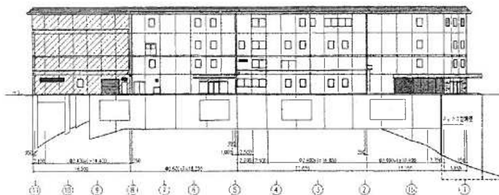
断面図 1:200
